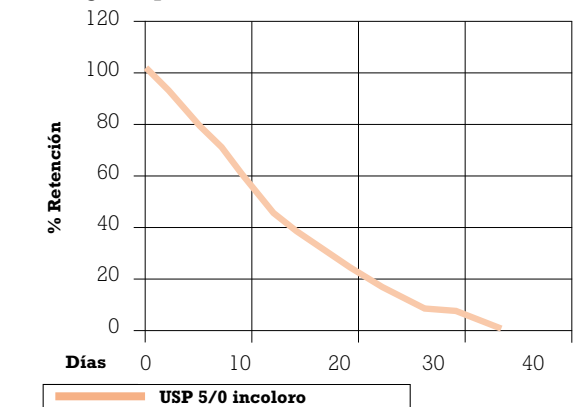
Absorción in vitro Poliglicaprona incolora
