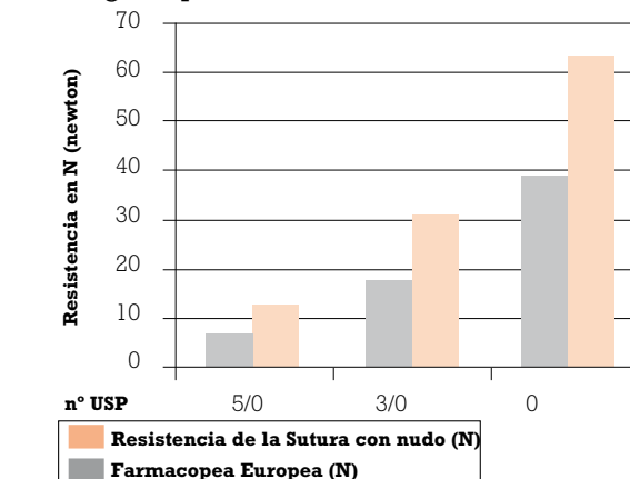
Resistencia a la rotura de la Sutura de Poliglicaprona violeta
